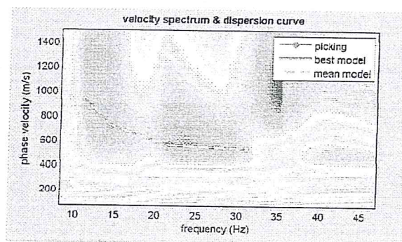
Figura 4: spettro di velocità tratto dalla prova MASW e relativo picking.
